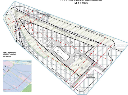
ПРОЕКТНИЙ ПЛАН ПОСІДНАНИЙ ЗІ СХЕМОЮ ПЛАНУВАЛЬНИХ ОБМЕЖЕНЬ М 1 : 1000
